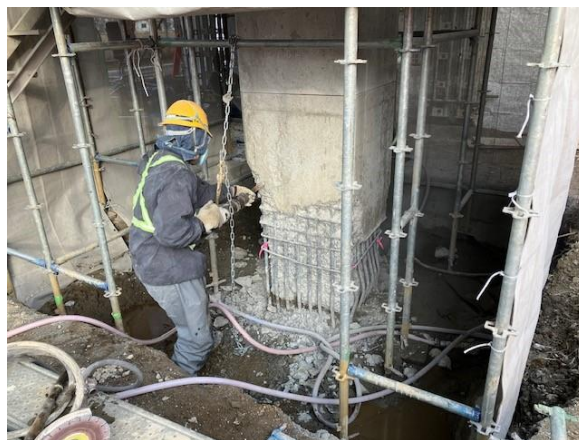
柱鉄筋修繕（12月17日撮影）
